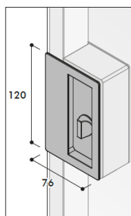
GEOD avec serrure à condamnation
