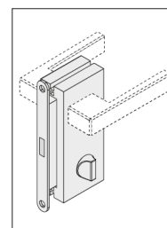
ZANTE VERTICALE avec serrure à condamnation
