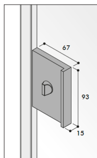
Serrure à condamnation
