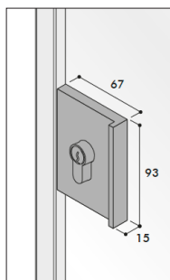
Serrure à clé
